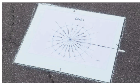
Figure 14. Gabarit utilisé pour la construction de l'orbite de la planète naine Cérès dans la cour de l'INSPE de Lille. Le gabarit est placé en respectant la position du centre et la direction de l'axe vernal grâce au rectangle et la flèche tracés à la craie. Il s'agit d'une représentation réduite du planétaire humain à construire.
