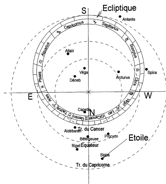
Figure 21. L'araignée de l'astrolabe.
