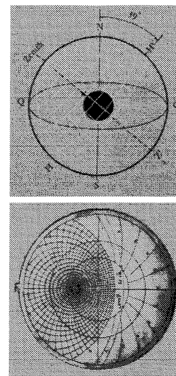
Figure 19. Almucantarats et cercles d'égal azimuth pour un lieu de latitude 39° ; tympan correspondant (tiré de The Planispheric Astrolabe , National Maritime Museum, Greenwich).
