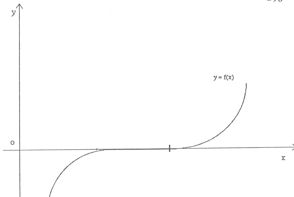
figure 3 : une fonction très voisine de f (pour la norme uniforme) peut avoir un zéro unique très éloigné de celui de f
