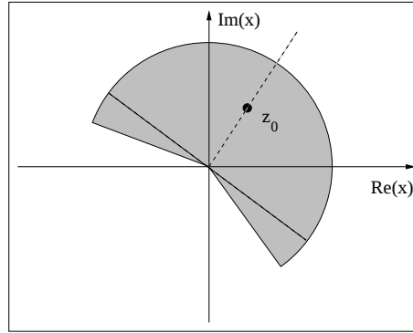
FIG. 2 – Un secteur d'analyticit  de la transform e de Laplace dans une direction qui n'est pas une direction de Stokes
