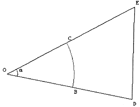
FIG 4 : Le triangle plan OED
