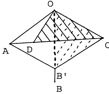
FIG 19 : Le tétraèdre OAB'C
