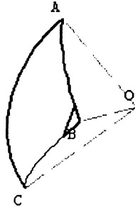
FIG 15 : Quatrième cas de résolution de triangle sphérique
