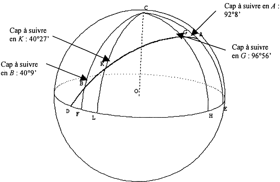
FIG 4 : Le triangle sphérique DKL
