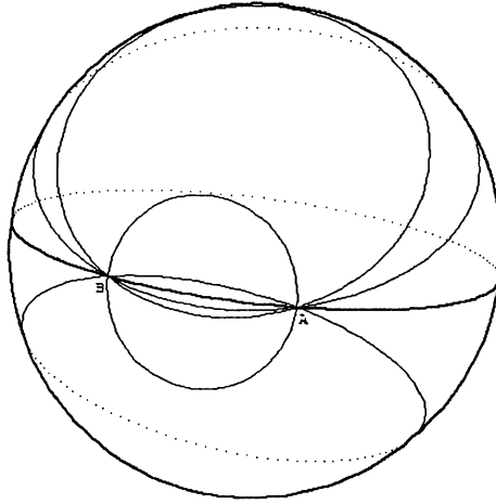
FIG 5 : Exemples de chemins circulaires reliant A à B , dont celui de diamètre [AB]
