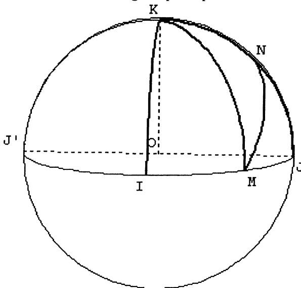
FIG 8 : Les triangles sphériques de l'exemple
