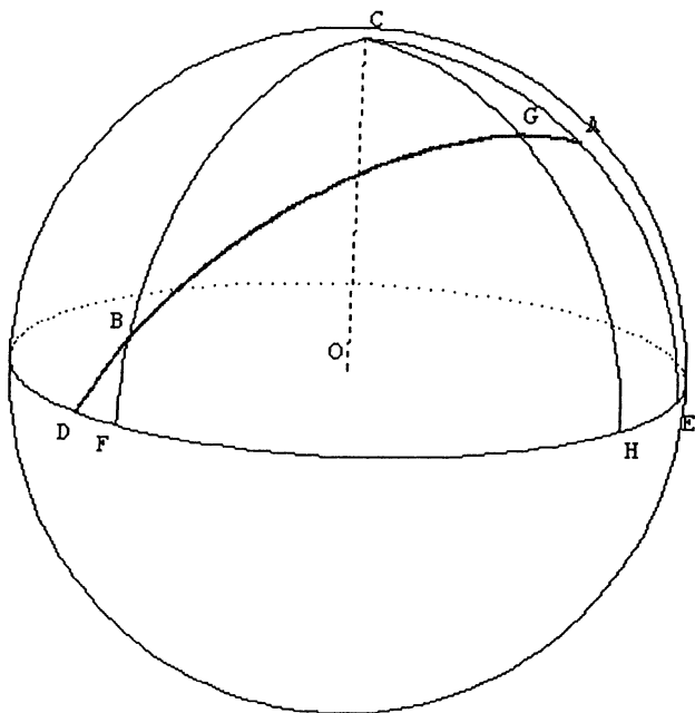
FIG 3 : Le cours droit de A vers B
