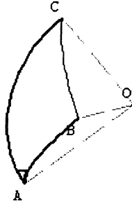
FIG 11 : Premier cas de résolution de triangle sphérique
