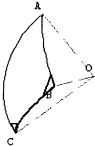
FIG 13 : Deuxième cas de résolution de triangle sphérique
