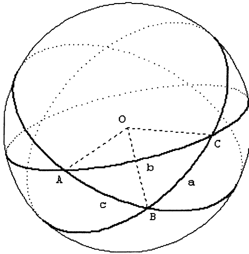
FIG 18 : Le triangle sphérique ABC avec b > a
