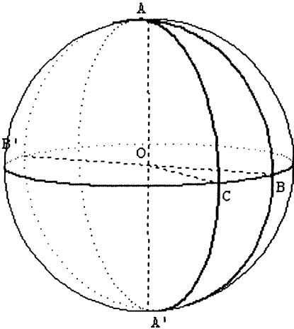
FIG 8 : Le triangle sphérique ABC avec deux côtés et deux angles droits
