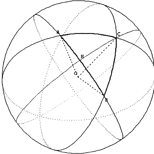
FIG 17 : La hauteur CH intérieure au triangle ABC et à son supplémentaire ABC'
