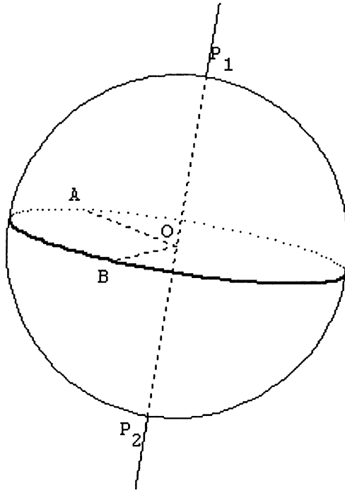
FIG 4 : L'axe polaire ( P_1P_2 ) du grand cercle contenant A et B
