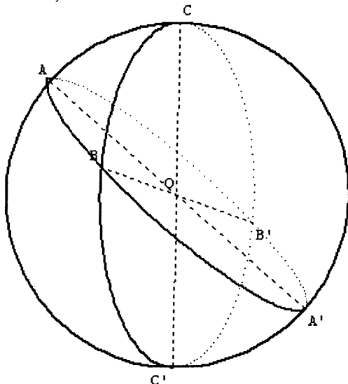
FIG 20 : La demi-sphère visible se décompose comme un puzzle
