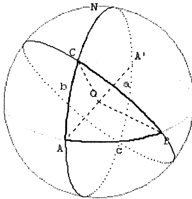
FIG 16 : Le triangle sphérique ABC rectangle en A
