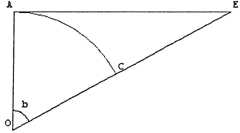
FIG 3 : OAE rectangle en A
