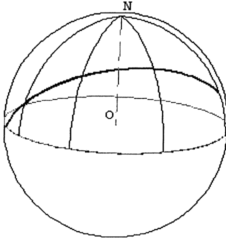
FIG 5 : Intersection du cours droit et des méridiens
