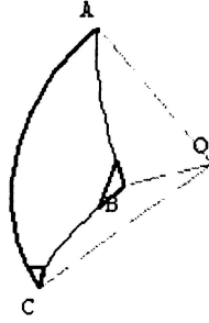
FIG 14 : Troisième cas de résolution de triangle sphérique
