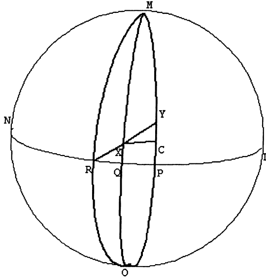
FIG 7 : Les triangles RXQ et XCY définis par le quatrième rumb RY ( 45^\circ )
