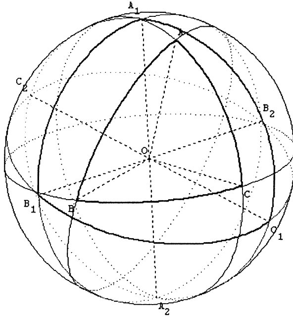
FIG 14: Le triangle sphérique ABC et son triangle sphérique polaire associé A_1B_1C_1 3
