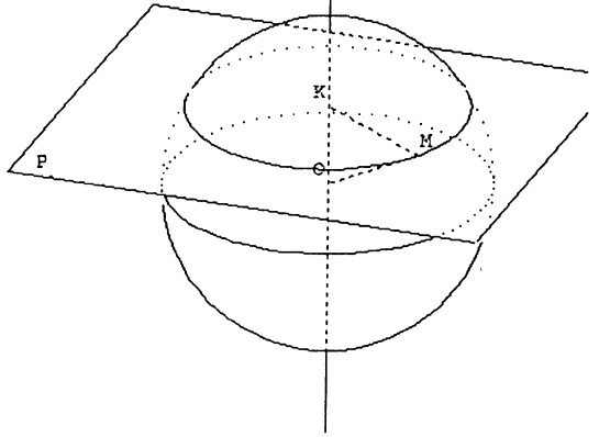
FIG 1 : Intersection d'un plan et d'une sphère
