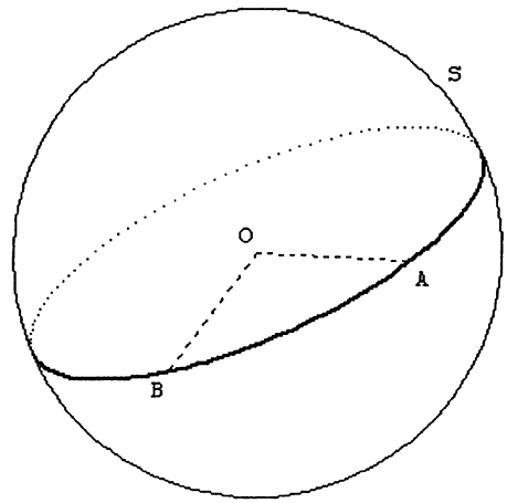
FIG 3 : Un seul grand cercle contient A et B non diamétralement opposés
