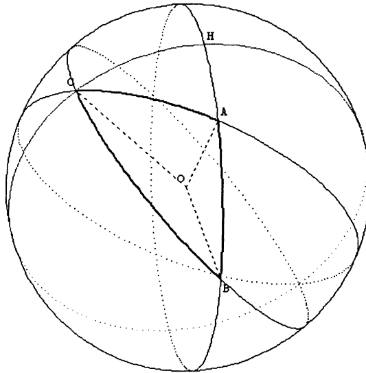
FIG 18 : La hauteur CH extérieure à ABC
