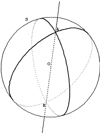
FIG 2 : Grands cercles de diamètre [AB]
