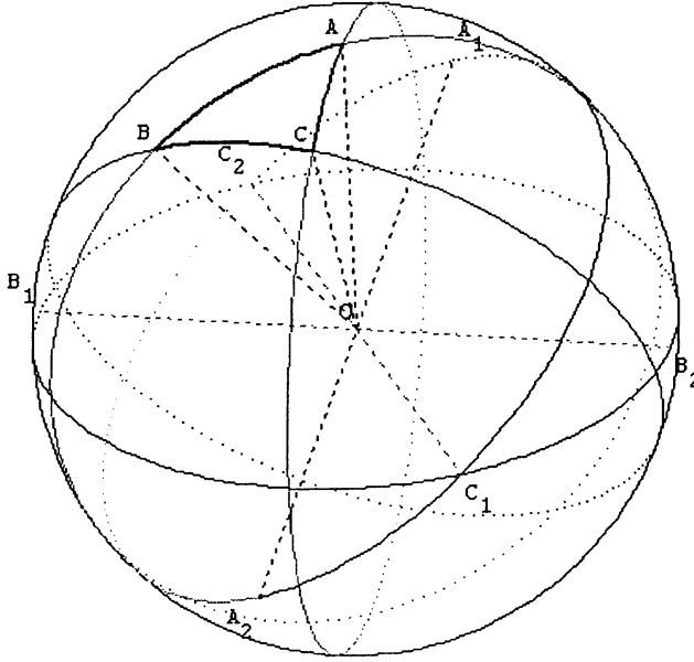
FIG 13: Le triangle sphérique ABC et les pôles A_i et B_i 2
