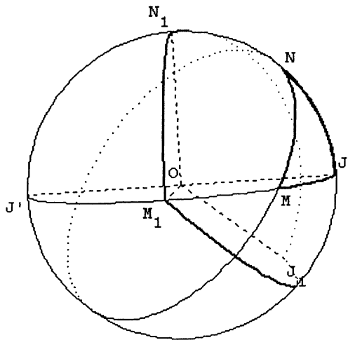
FIG 15 : Le triangle sphérique MNJ et son polaire
