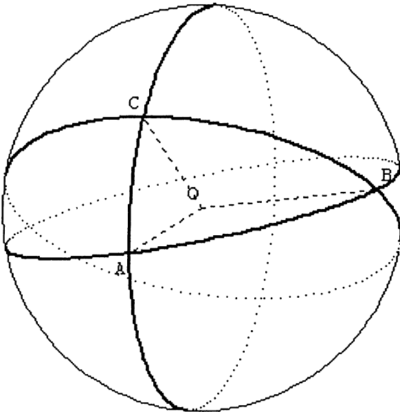
FIG 7 : Le triangle sphérique ABC
