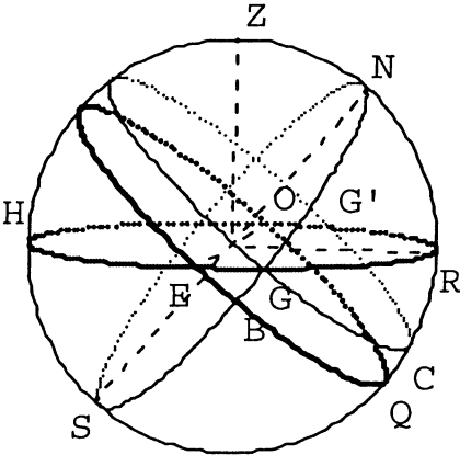
FIG 8 : Lever et coucher du soleil
