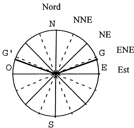
FIG 9 : Le cercle horizon de l'observateur
