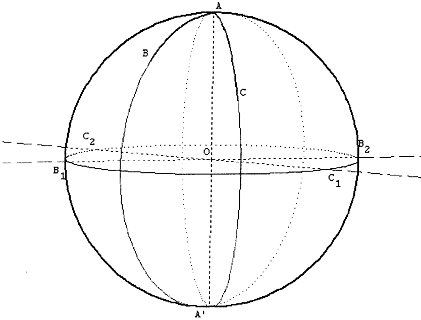
FIG 12 : Les axes polaires (B_1B_2) et (C_1C_2) des grands cercles AC et AB
