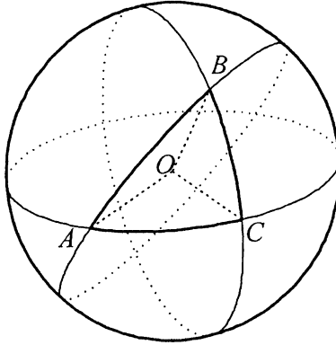
FIG 10 : Les angles et les côtés du triangle sphérique ABC
