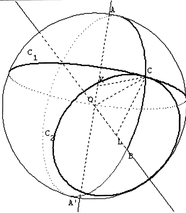
FIG 6 : Le grand cercle AB et les deux petits cercles C_1 et C_2
