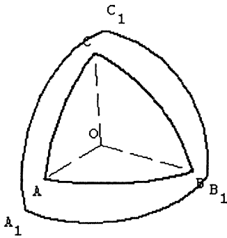
FIG 12 : Les triangles sphériques ABC et A_1B_1C_1 polaires l'un de l'autre
