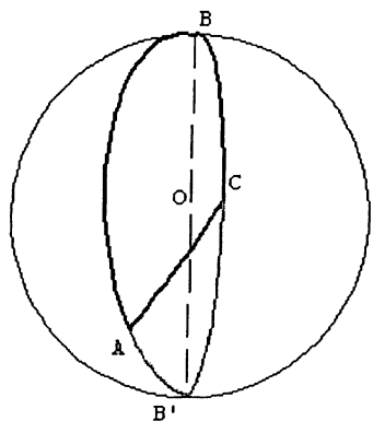
FIG 6 : Les triangles sphériques ABC et AB'C
