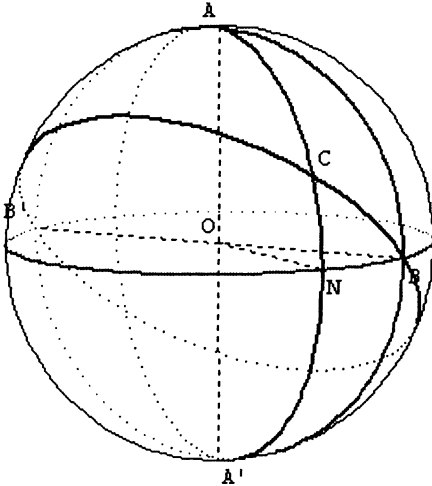
FIG 9 : Le triangle sphérique ABC avec un côté droit
