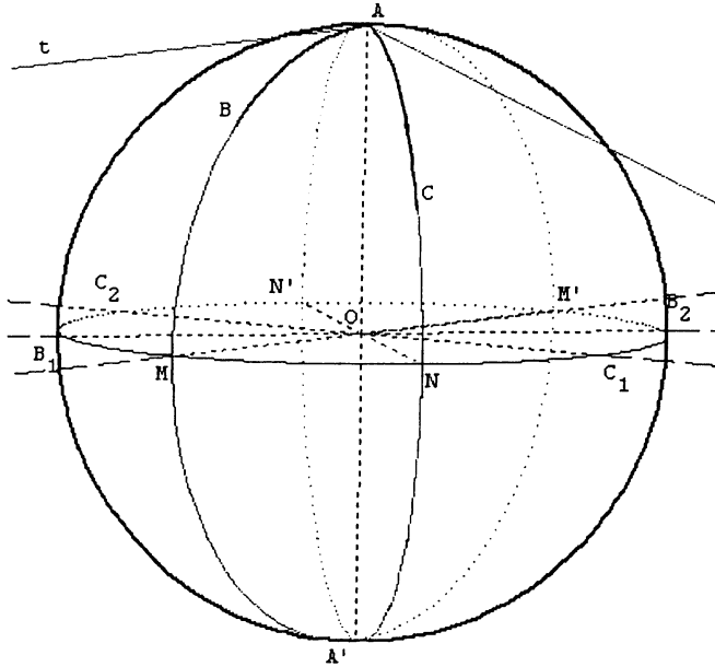
FIG 16 : Les grands cercles AB et AC , leurs axes polaires et leurs demi-tangentes
