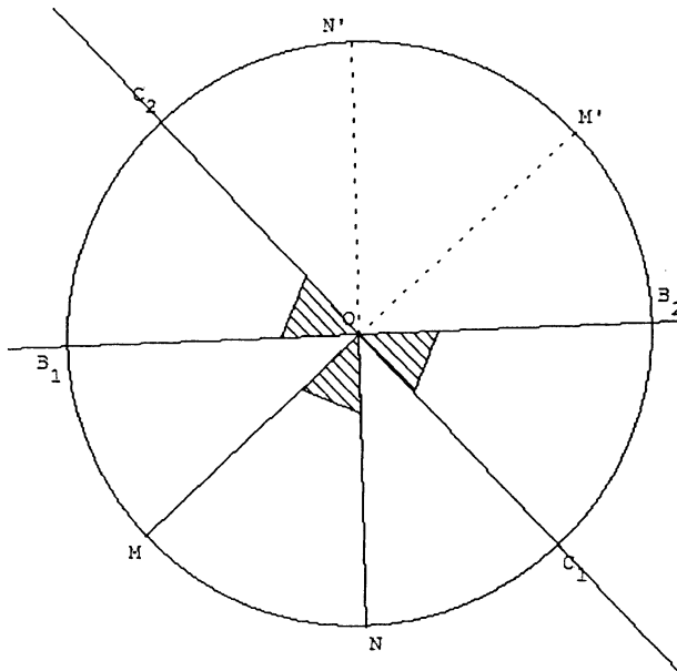
FIG 17 : Section de la sphère par le plan du grand cercle B_1B_2C_1C_2
