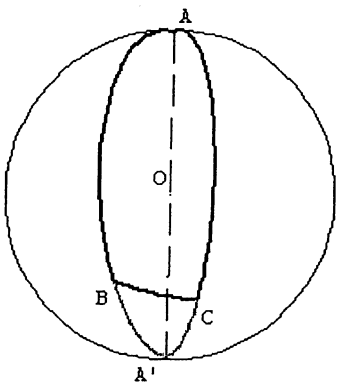
FIG 7 : Les triangles sphériques ABC et A'BC
