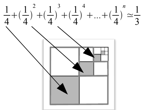
Image 2 - Une interprétation géométrique de l'expression arithmétique-algébrique donnée.
