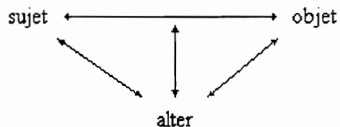
fig. 3 - Le schéma tripolaire caractérisant la médiation
