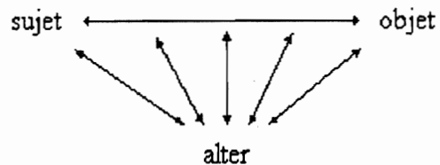
fig. 4 - Les différentes formes de médiation
