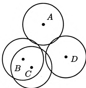
Pas de zone commune
