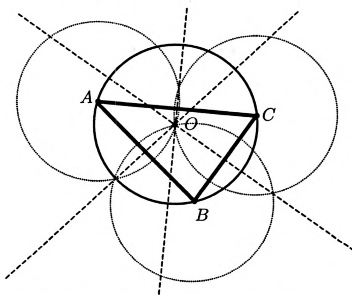
Le cercle circonscrit, meilleure solution.
