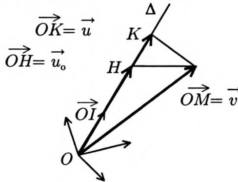
Dessin dans un hyper-espace de dimension n
