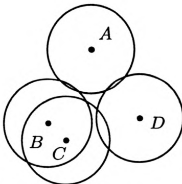
Pas de zone commune
