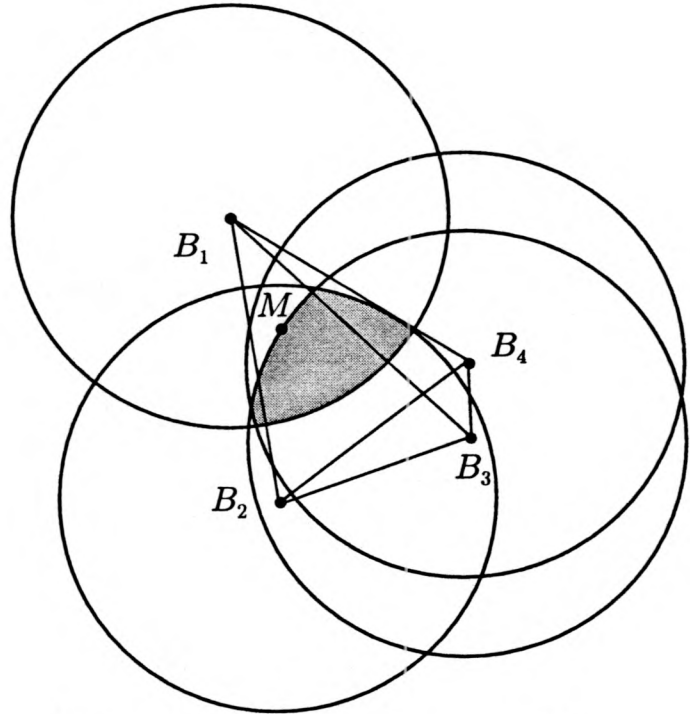
La ligne de niveau qui passe par M
