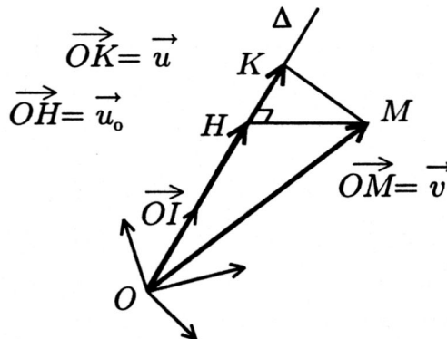
Projection dans un hyper-espace de dimension n
