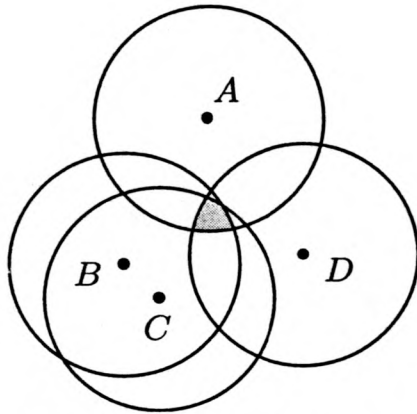
Il y a une zone commune
