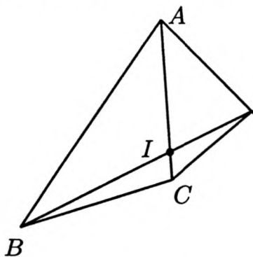
Quadrilatère convexe
