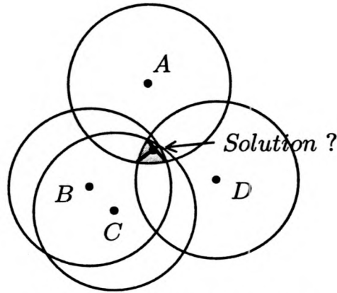
Proposition pour le centre
