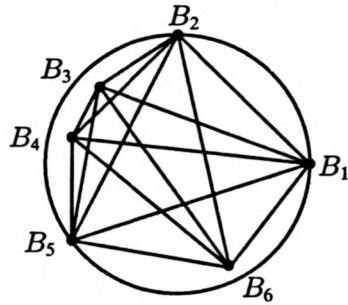
Exemple de solution cas n°1
