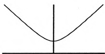
allure de f_i , c_i \neq 0
