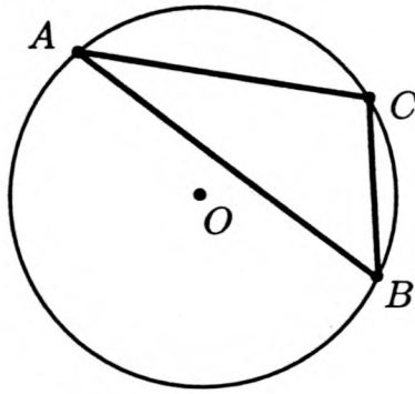
2 ème triangle (le cercle circonscrit)
