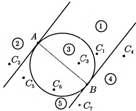
Dessin n°1 bis
