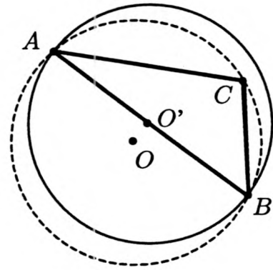
2 ème triangle (la solution)
