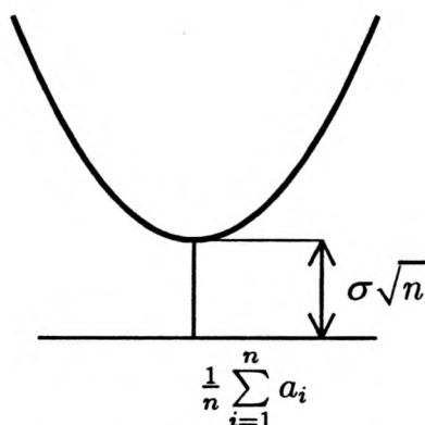
Allure de la courbe représentant \phi
