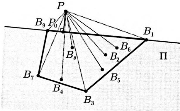
Le projeté est sur un côté
