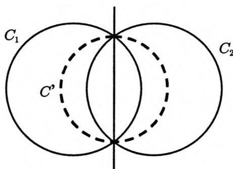
Unicité de la solution
