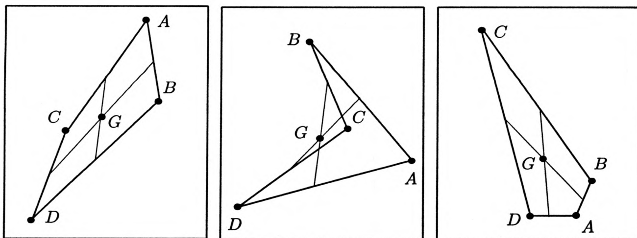
Étude de centres de gravité...
