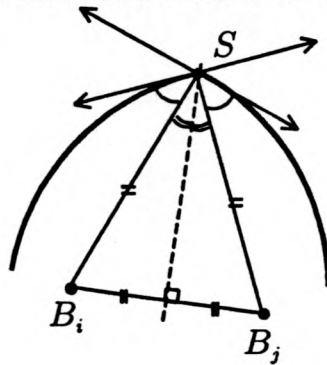
Sommet, centres, tangentes, bissectrice
