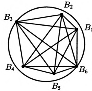
Exemple de solution cas n°2
