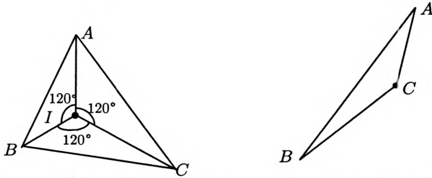
Pas de centre de Toricelli ici
