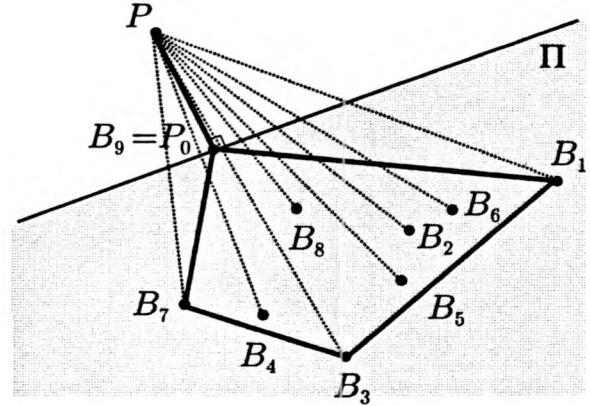
Le projeté est un sommet
