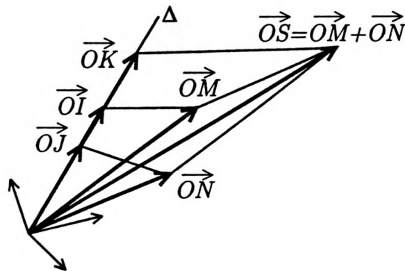
Somme de deux séries statistiques
