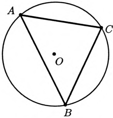
1 er triangle
