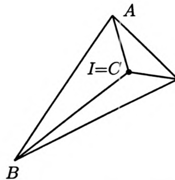
Quadrilatère non convexe
