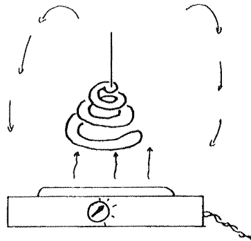
L'air chaud s'élève au-dessus de la plaque chauffante et redescend à la périphérie (ce qu'on a du mal à montrer expérimentalement).
