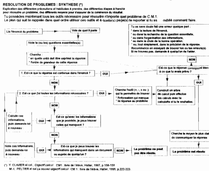
FIGURE 1 — Un algorithme de résolution enseigné au CM1
