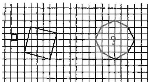
exemples de polygones à 4 et 8 côtés
