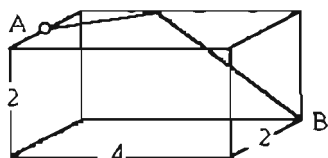
fig. 5 : quel est le plus court chemin de A à B ? fig. 6 : ceci n'est PAS une pyramide tronquée, pourquoi ?
