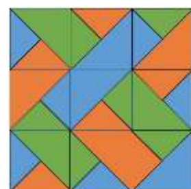
Un carré obtenu en manipulant les dessins de seize pièces
