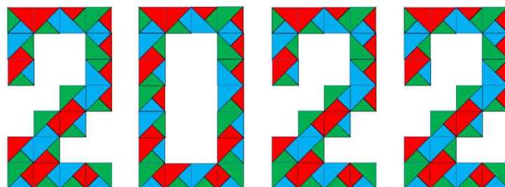
(carrés de MacMahon « du Caire »)
