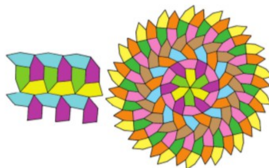
2. L'UNIQUE PENTAGONE dont les angles vérifient les relations A + 2B = C + 2E = A + C + 2D = 360^\circ permet de construire plusieurs pavages différents, périodiques (comme ci-dessus à gauche) ou non (comme ci-dessus à droite).
