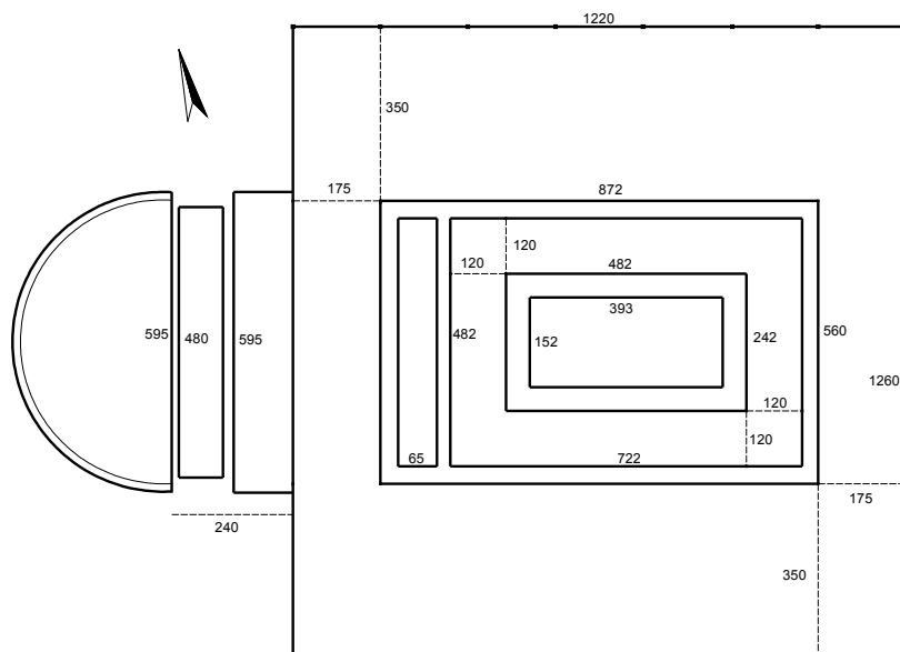
Figure 2. Dimensions en cm.
