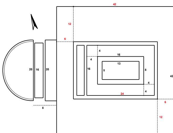
Figure 3. Dimensions en pieds (pied faible en rouge, pied fort en noir)
