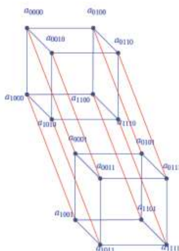
Figure 3 – L’hypercube et le codage binaire de ses sommets.
