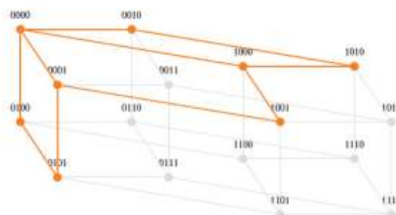
Figure 4 – Le codage de Zeckendorf sur l’hypercube. Les points en orange sont ceux pour lesquels le codage n’a pas deux 1 consécutifs.
