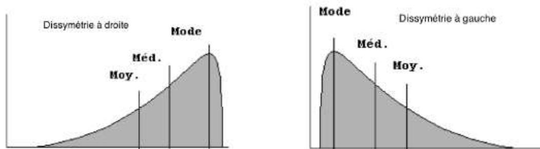
Figure 1 -Distributions dissymétriques
