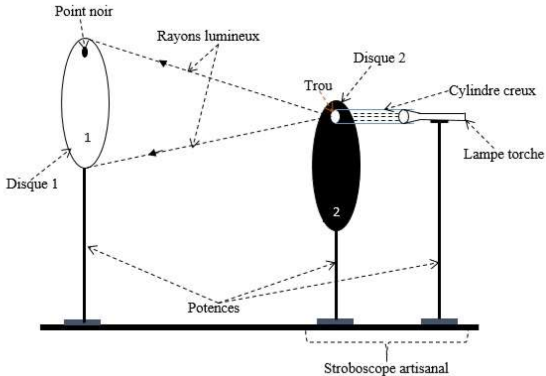
Figure 1 : Dispositif expérimental
