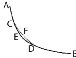
Figur 4.10: Kurven ACEDB er den hurtigste rute som et punkt med tyngde følger fra A til B.
