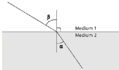
Figur 4.3: En lysstråle afbøjes ved normalen, der står vinkelret på overgangen mellem to medier med forskellige densiteter. Lysstrålens indfaldsvinkel er \beta og brydningsvinklen er \alpha
