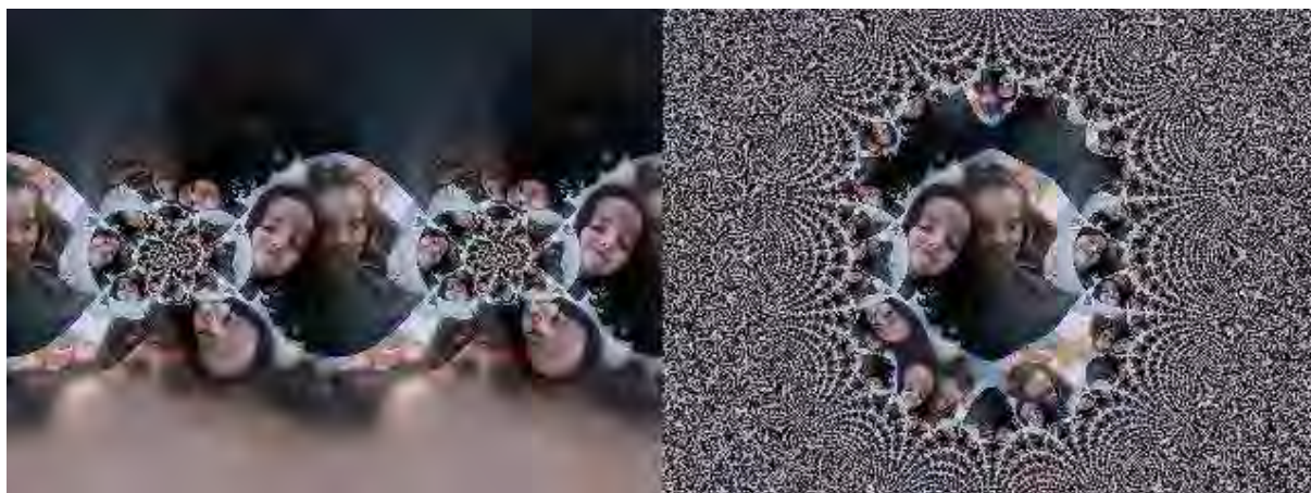
Figure 4 – La comparaison entre la fonction tangente et son développement en polynôme de Taylor permet de rendre visuel la notion de disque de convergence dans lequel la série converge vers la fonction (la différence entre les deux images y est très faible) et en dehors duquel elle diverge
