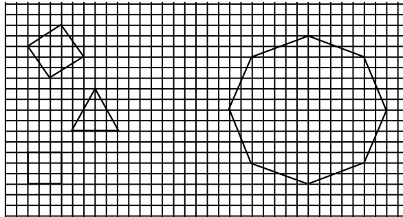
Figure 2 – Polygones à sommets entiers
