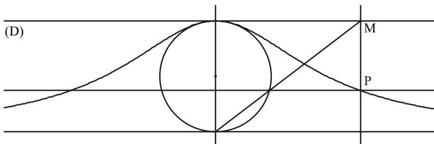
Construction : quand le point M décrit la droite (D), le point P décrit la cubique d'Agnesi.
